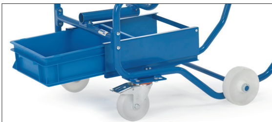
Cuvette de réf. 2019 Kit pour berceau 2015 et 2016. Cuvette en plastique de 12 litres de contenance.
