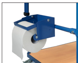
Porte-rouleau de papier absorbant. Kit pour servantes prévu pour un rouleau de diamètre et largeur de 210 mm. Détails voir page 193.
